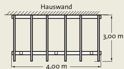
Planungsbeispiel einer Pergola ohne Pergolaverbinder
